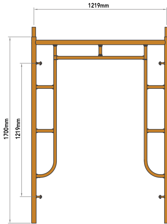
BEATTY FRAME
